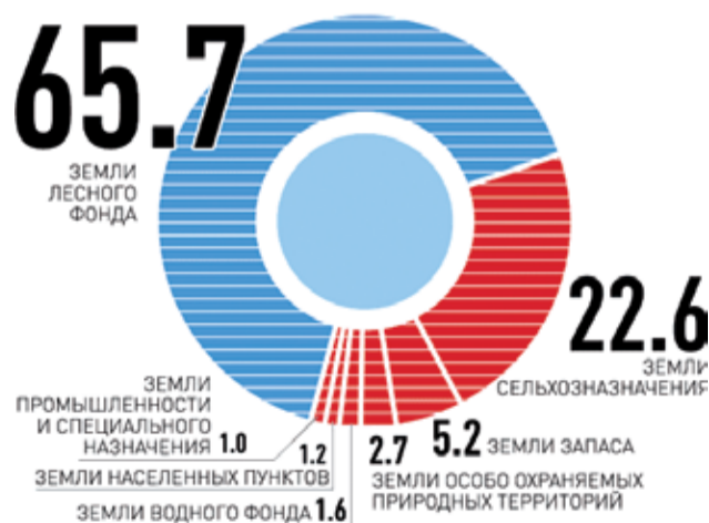
РАСПРЕДЕЛЕНИЕ ЗЕМЛИ В РОССИИ ПО КАТЕГОРИЯМ, % (НА 1 ЯНВАРЯ 2014 ГОДА)
