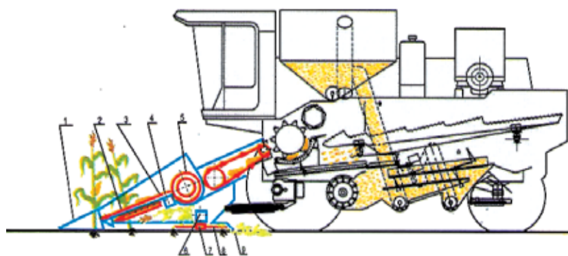
Технологическая схема уборки кукурузы жатками КМС-6 и КМС-8
