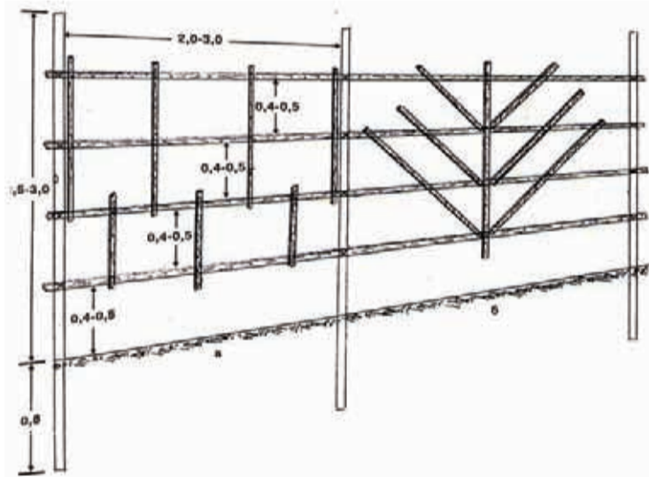
Рис.4 Устройство шпалер из реек: а) для двойной U-образной кроны; б) для трёхъярусной наклонной пальметты. Размеры реек: горизонтальные — 50x50 мм, вертикальные — 50x25 мм. Размеры в метрах
